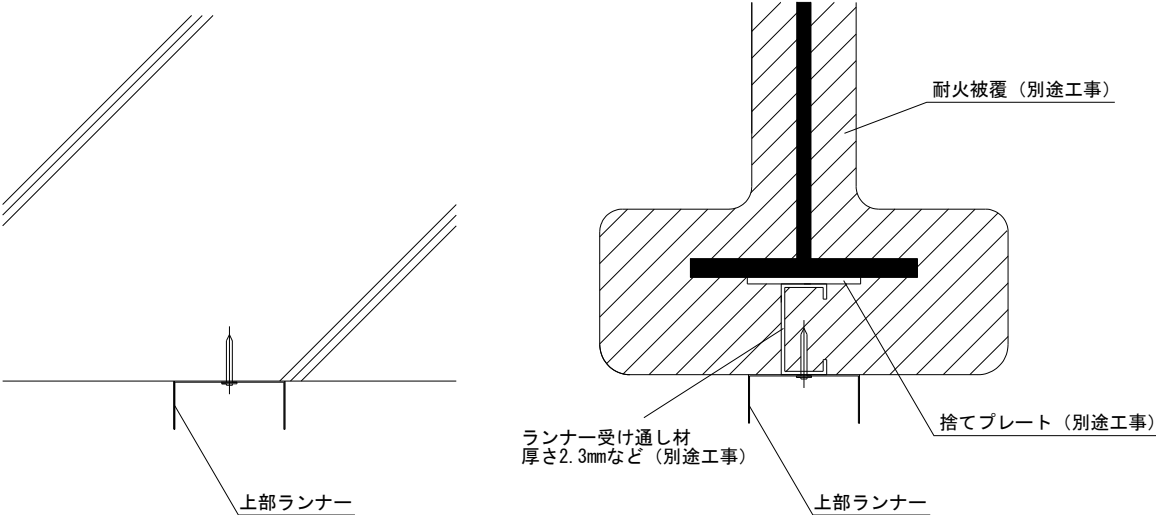
<天井スラブおよびRCへのランナーの取り付け例> <鉄骨梁へのランナーの取り付け例>
