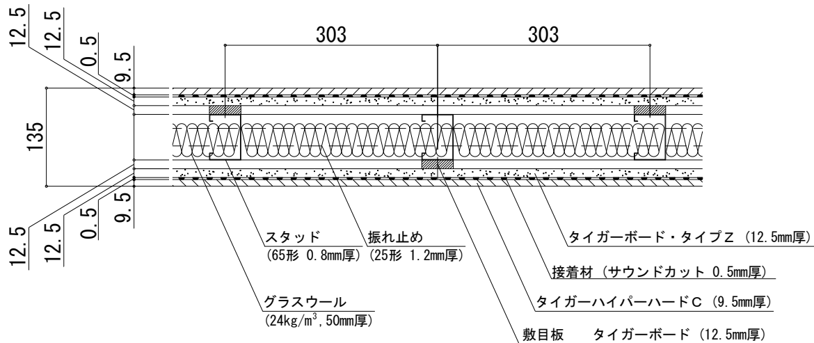
水平断面図（「ハイパーウォールZ・WI 敷目板タイプS（生活音対策）仕様」遮音測定時（S－252－30参照）の壁構造）
