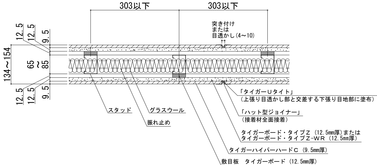
水平断面図 (「ハイパーウォールZ・WI 敷目板タイプ 目透かし仕様」壁構造の仕様)
