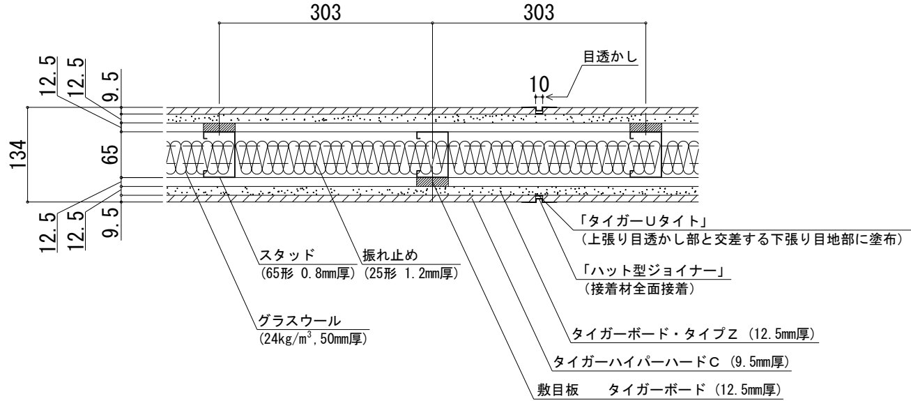
水平断面図 (「ハイパーウォールZ・WI 敷目板タイプ 目透かし仕様」遮音測定時 (S-252-31参照) の壁構造)
